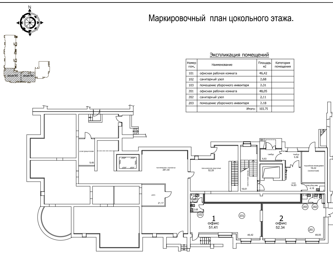
Маркировочный план 1 этажа.
