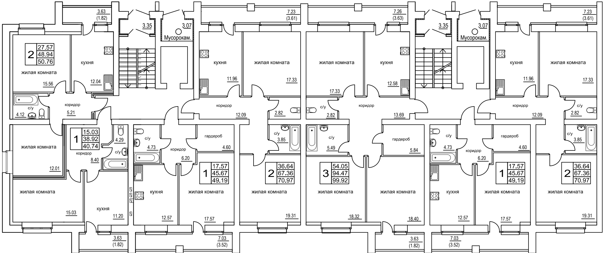
Маркировочный план 1 этажа.
